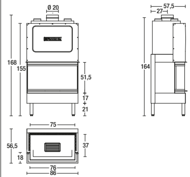
Model: 700 HT/B
