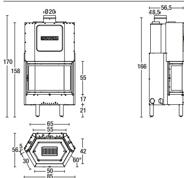
Model: 750 HT/B
