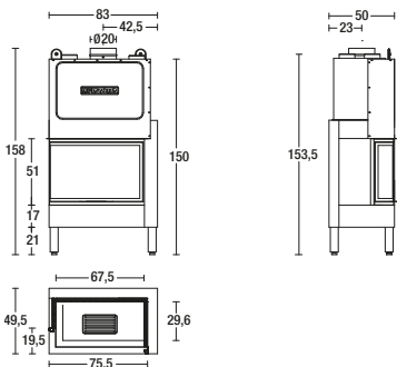
Model: 810 HT/A
