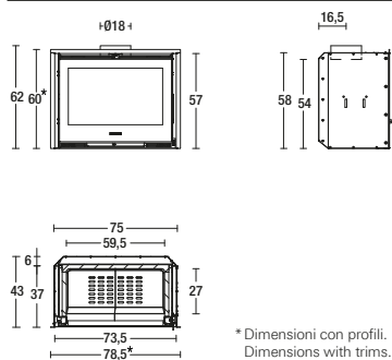
Model: IL 75/58
