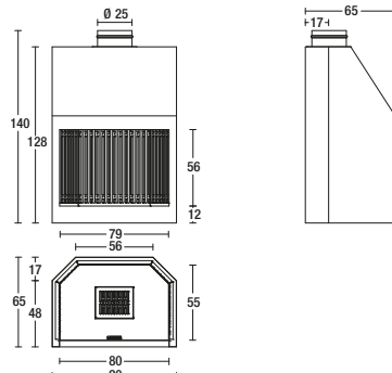
Model: MA 261
