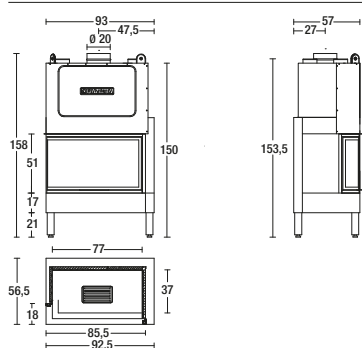
Model: 801 HT/A
