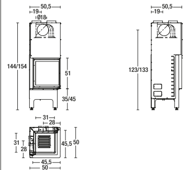
Model: 510 SL
