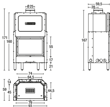
Model: 610 HT/B
