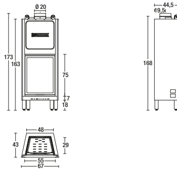
Model: 650 HT
