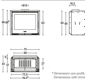
Model: IL 75/64
