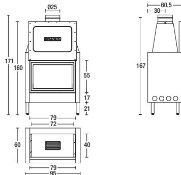
Model: 2010 HT/B
